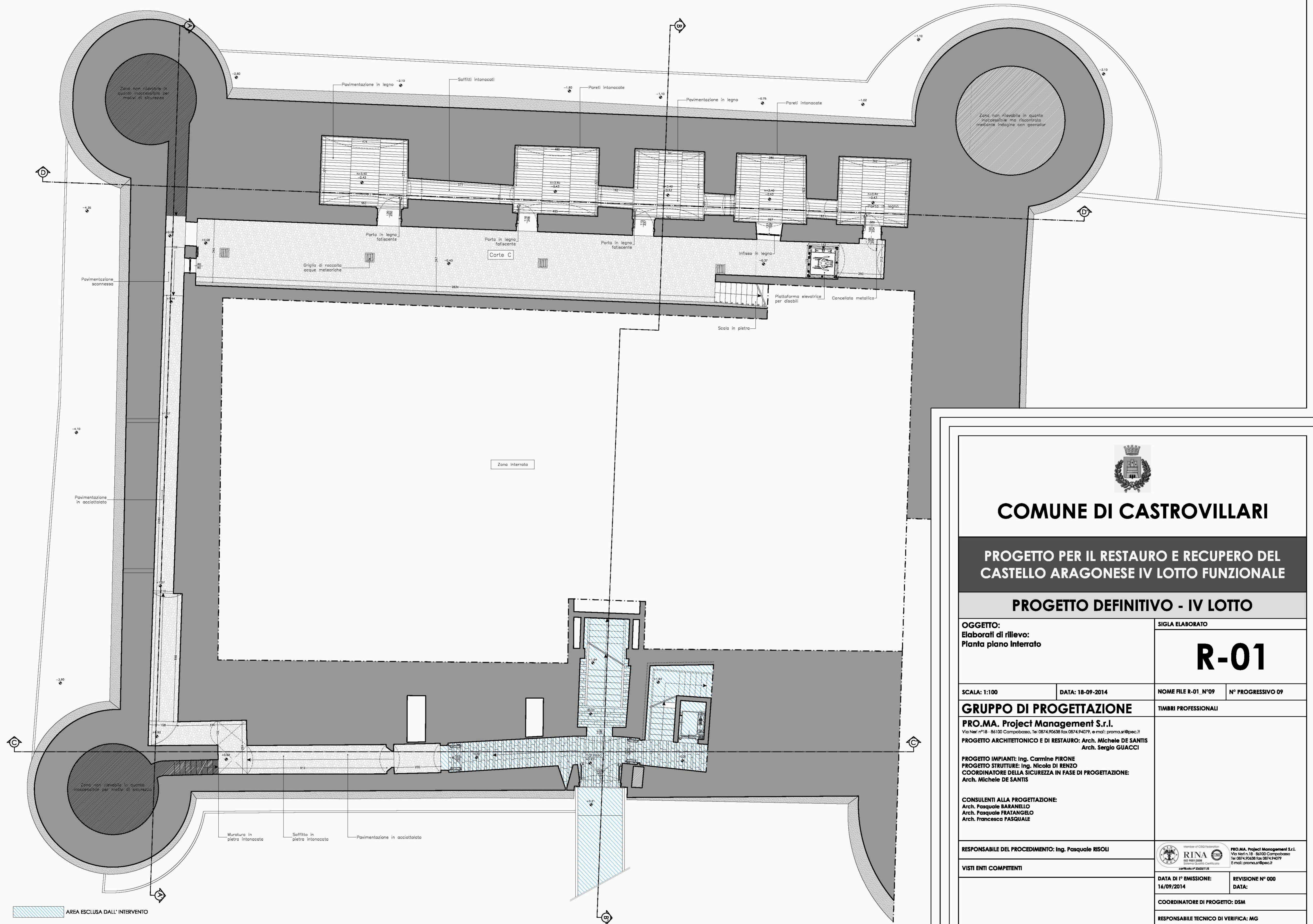
Pianta piano interrato - Sc. 1:100
